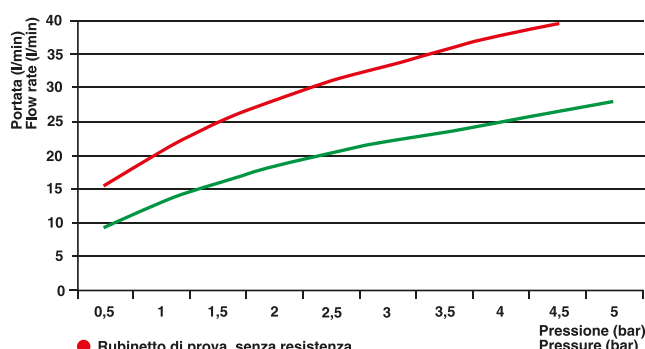
Curve di portata Flow rate curves
